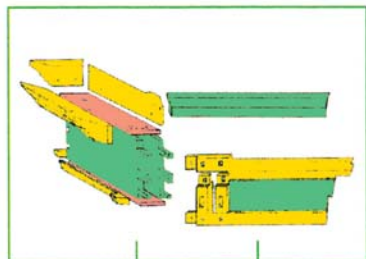
Egituraren xehekapena Desglose de la estructura
